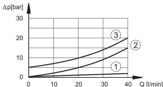
PERDITE DI CARICO \Delta p - Q
